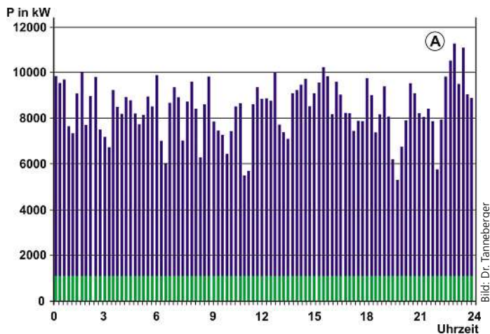
Bild 1: Das Diagramm zeigt den Leistungsverlauf einer Ofenanlage in einer Härtereie mit Leistungsspitzen ohne Padicon.
